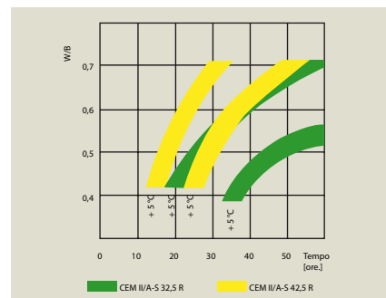
Tempo necessario per raggiungere la resistenza al gelo del calcestruzzo. (resistenza a compressione > 5 MPa in relazione al rapporto acqua/cemento con diverse temperature del calcestruzzo e diversi tipi di cemento)
