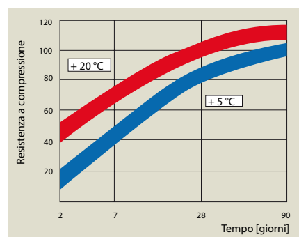
Evoluzione della resistenza a compressione del CLS (con CEM I 42,5 N) in funzione della temperatura del CLS
