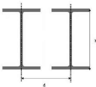
Figura C3.3.28 – Travi parallele
