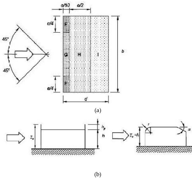
a) Suddivisione delle coperture piane in zone di uguale pressione, b) Altezza di riferimento per coperture piane con parapetti o raccordi (curvi e piani)
