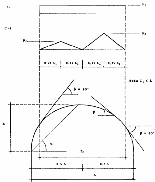
Fig C.6.6 - Coefficienti di forma per coperture cilindriche
