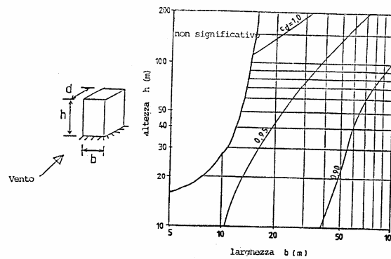
Fig. C.7.10 (a) - Edifici in c.a. o in muratura
