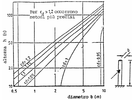
Fig. C.7.11 (b) - ciminere in acciaio, saldate, con rivestimento interno
