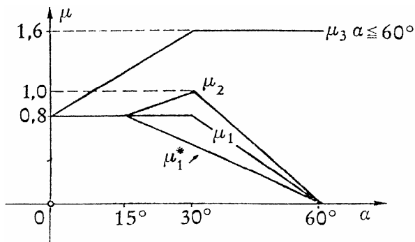
Fig. 6.2 - coefficienti di forma per coperture a falde
