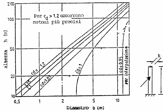
Fig. C.7.11 (a) - ciminere in acciaio, saldate, senza rivestimento interno
