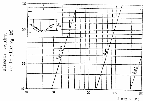
Fig. C.7.12 - Ponti stradali, ferroviari e pedonali
