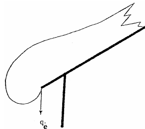
Fig. C.6.10 - Neve sporgente all'estremità di una copertura.
