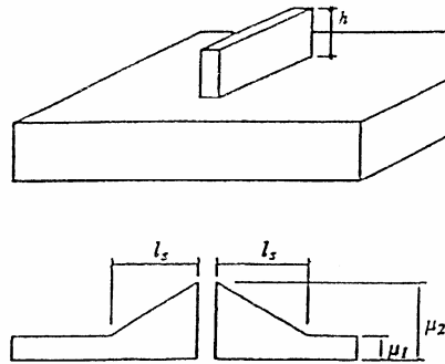
Fig. C.6.9 - Coefficienti di forma in corrispondenza di parapetti e pareti verticali.
