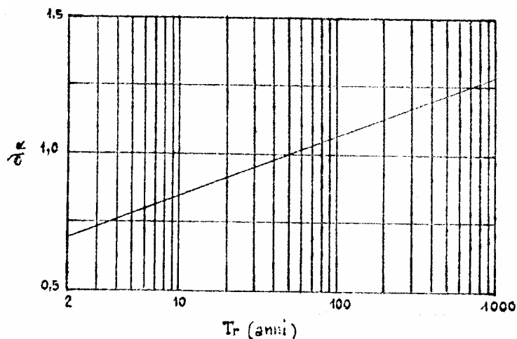
Fig. C.7.4 Valori dell'azione del vento in funzione dell'intervallo di ritorno.
