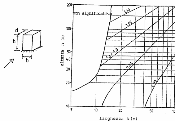
Fig. C.7.10 (b) - Edifici a struttura in acciaio
