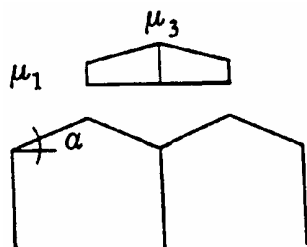
Fig. 6.5 - condizione ulteriore di carico per coperture a più campate. Particolare attenzione dovrà essere prestata per la scelta del coefficiente di forma \mu_3 quando una o entrambe le falde hanno inclinazione superiore a 60^\circ .
